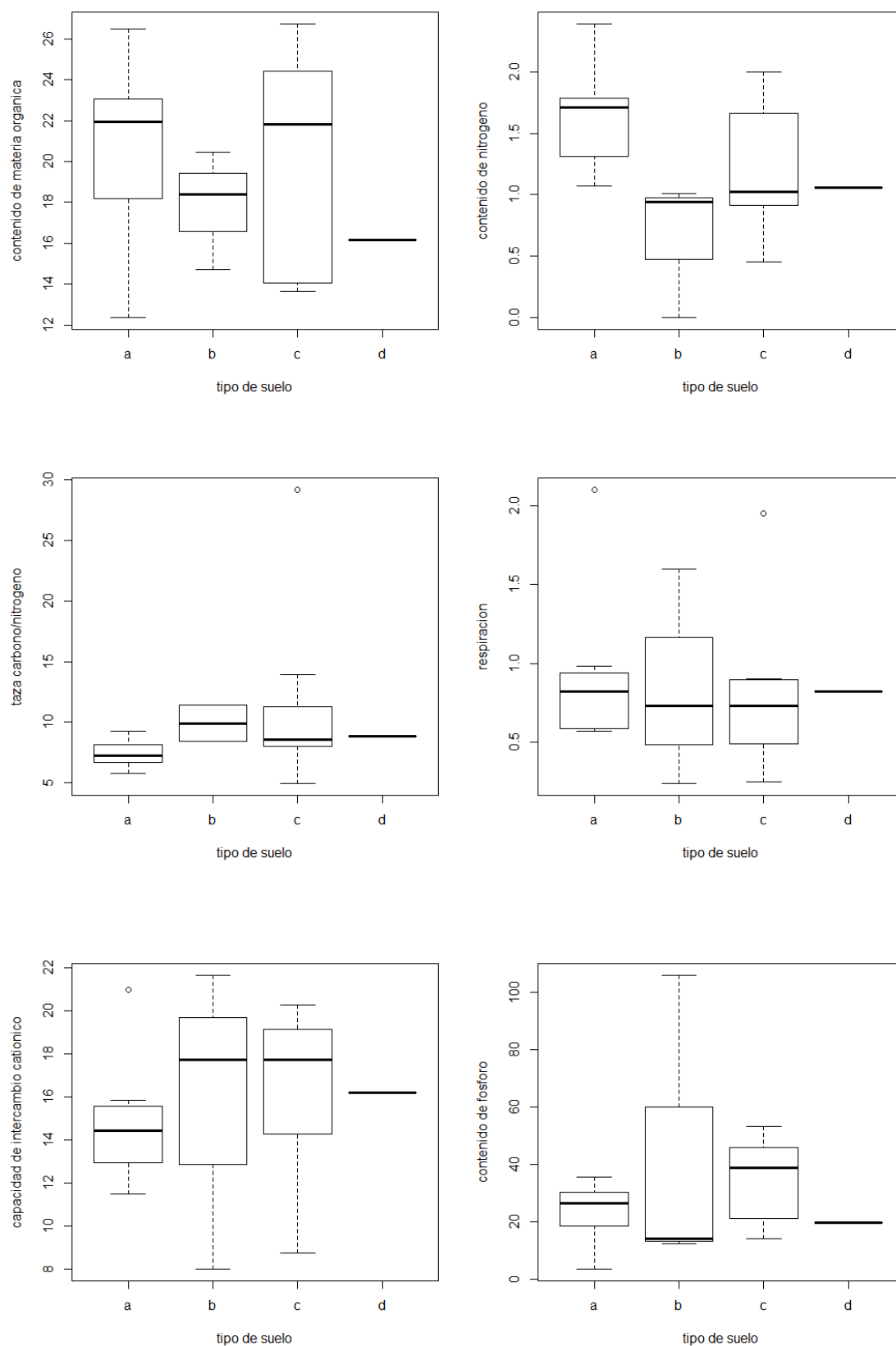
Ilustración 10: Efecto del tipo de suelo sobre los indicadores de fertilidad
