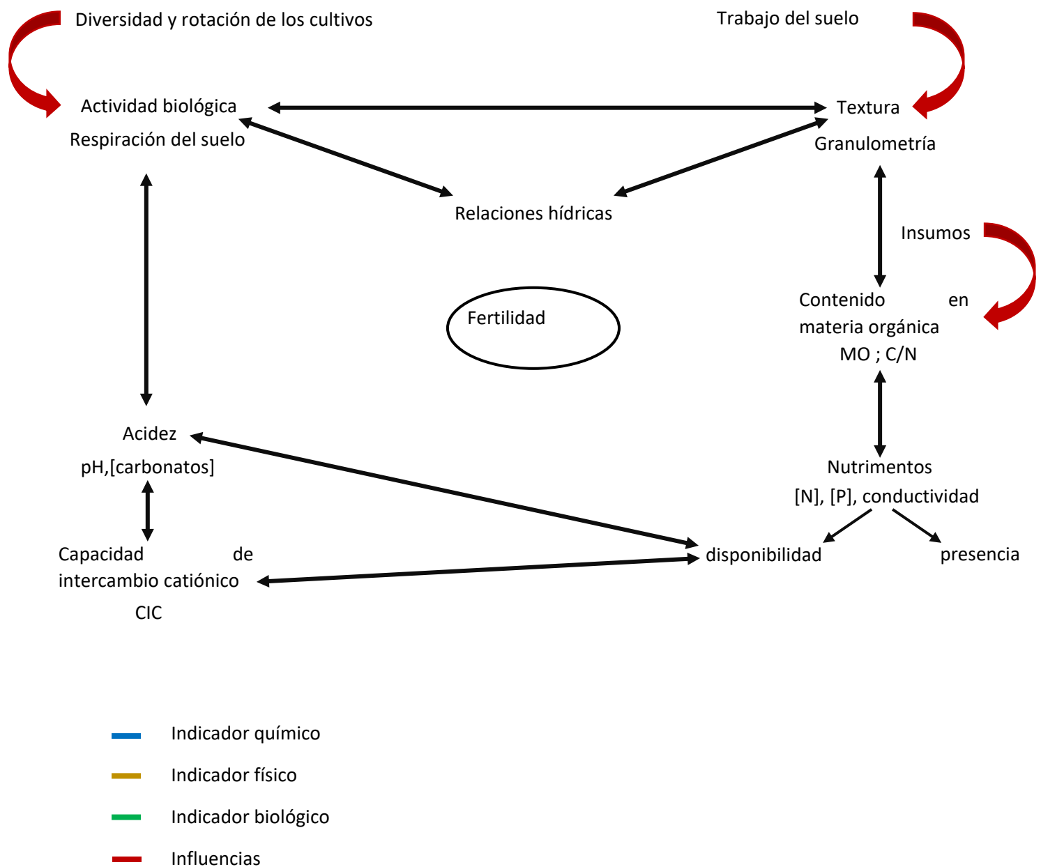
Ilustración 1: Interacciones en el suelo e indicadores correspondiendo
